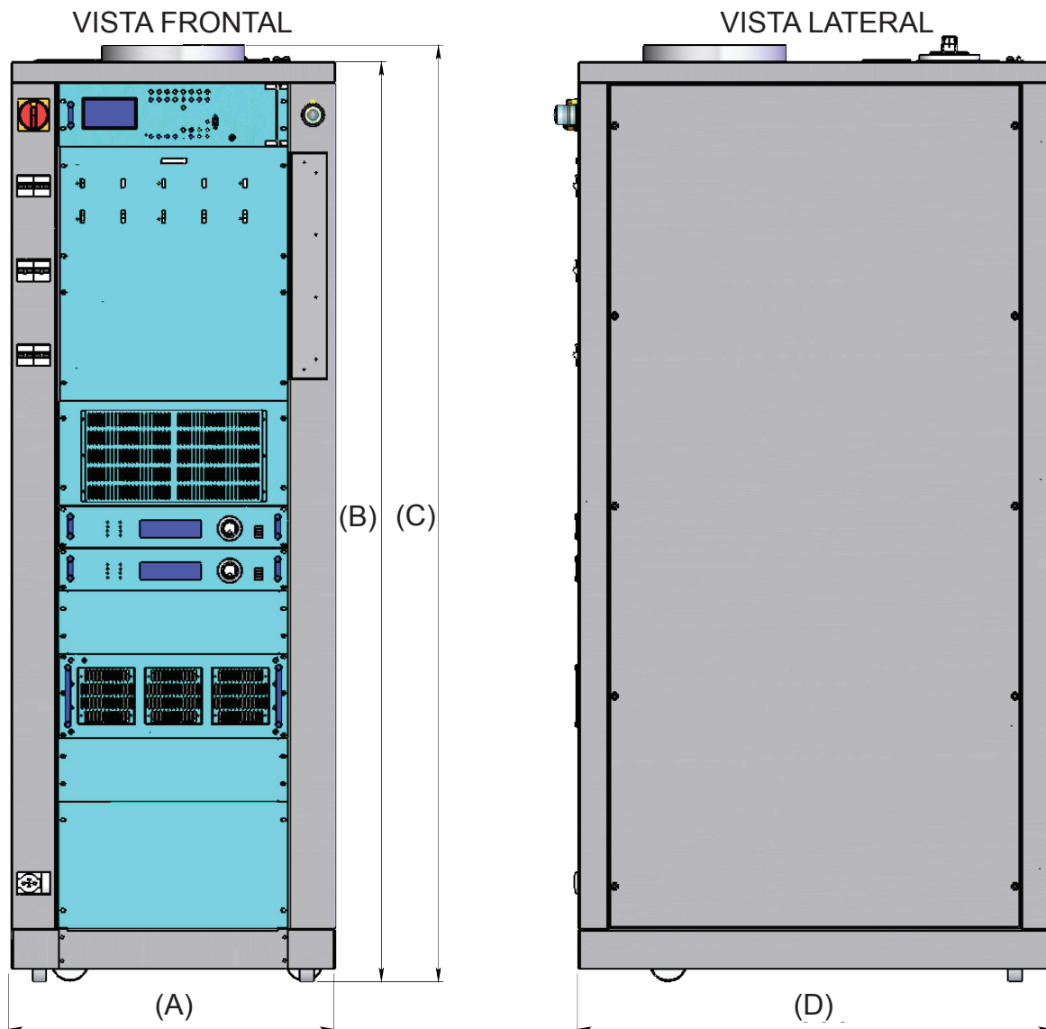
DIMENSIONES BASTIDOR
