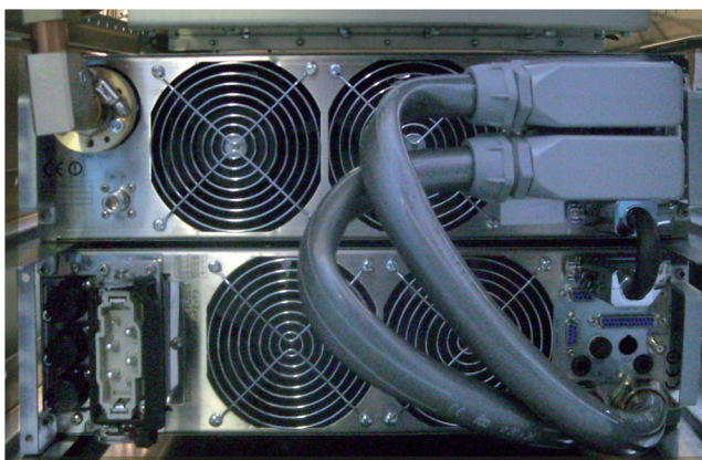
Figura 5-1 Esempio di installazione PJ5000U-K in rack
